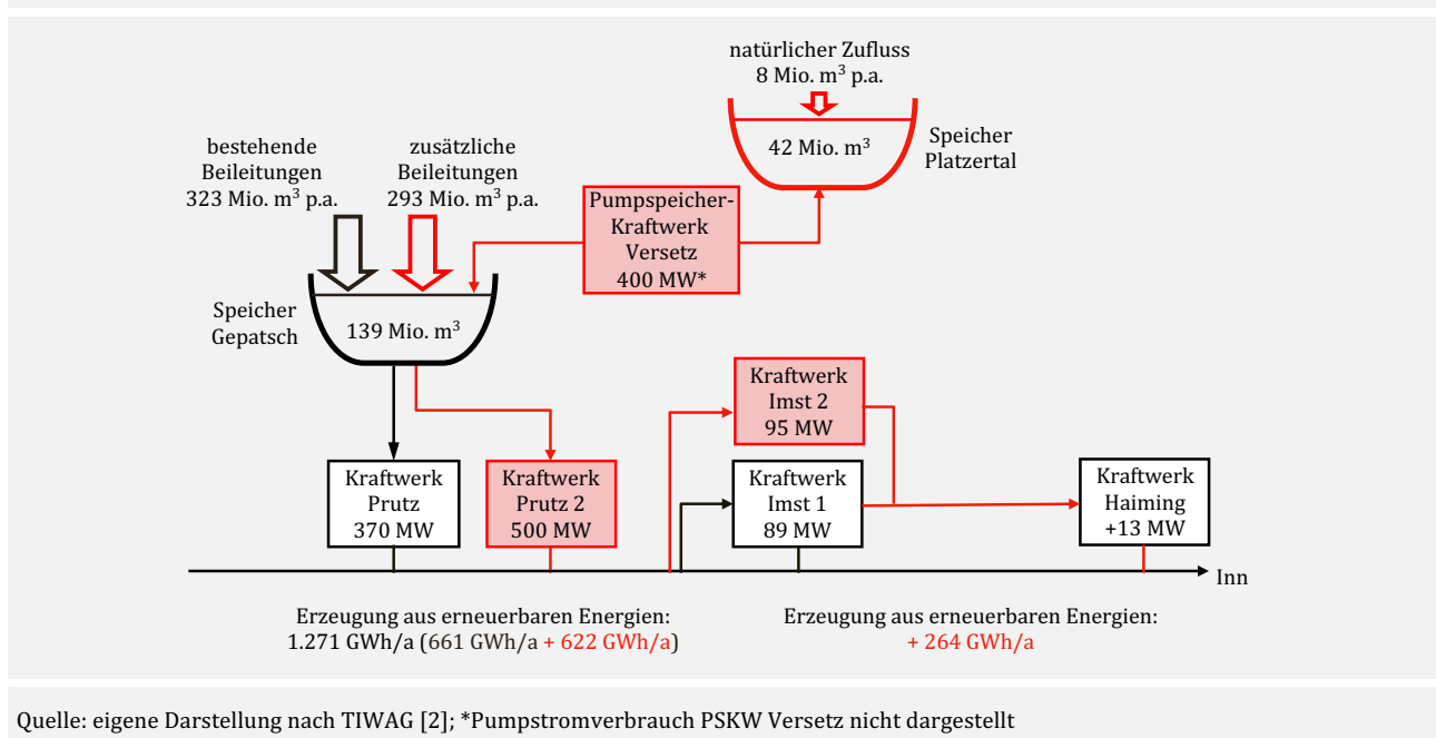
Abbildung 1: Schematischer Überblick Bestand und Ausbauvorhaben Kraftwerk Kaunertal
