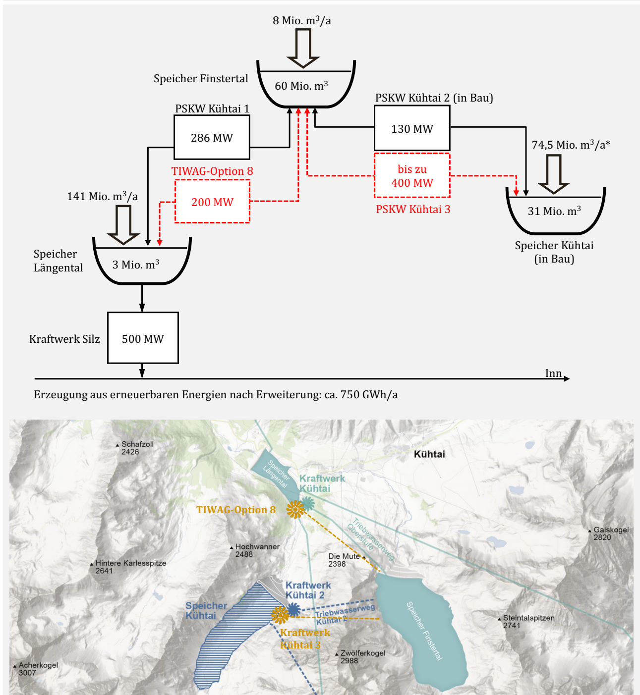
Abbildung 3: Schematischer Überblick (oben) sowie Projektübersicht (unten) der Kraftwerksgruppe Sellrain-Silz jeweils ergänzt um die Vorschläge für einen weiteren Ausbau der Pumpspeicherkapazitäten durch ein PSKW Kühtai 3 und/oder PSKW entsprechend TIWAG-Option 8
